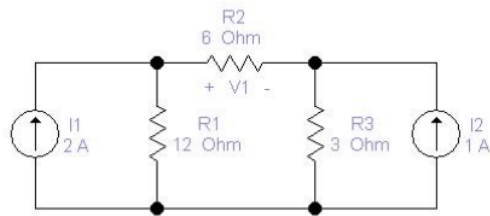
Gambar 4. Rangkaian Listrik dengan Sumber Arus
