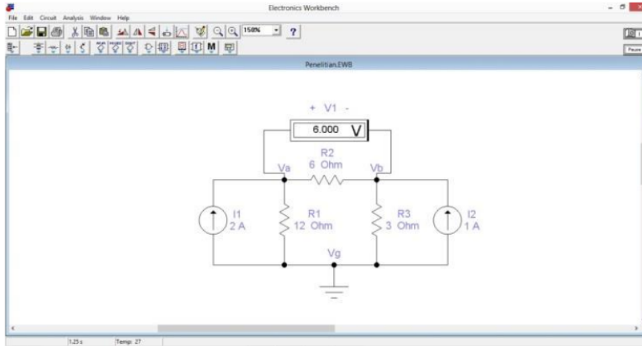
Gambar 8. Hasil Simulasi Analisis Node Rangkaian Listrik Menggunakan Software Electronics Workbench
