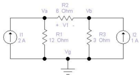
Gambar 5. Metode Analisis Node Pada Rangkaian Listrik
