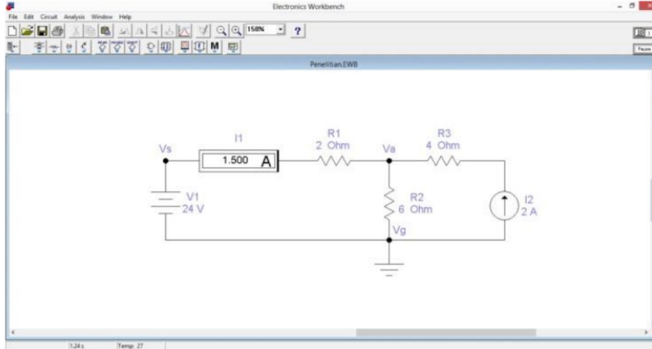
Gambar 12. Hasil Simulasi Analisis Supernode Rangkaian Listrik Menggunakan Software Electronics Workbench
