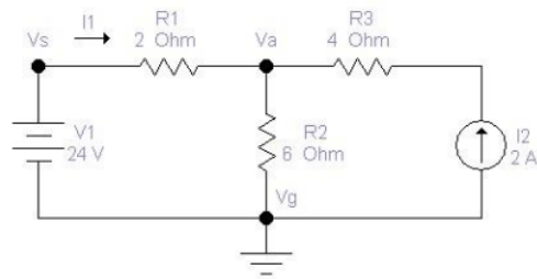
Gambar 10. Metode Analisis Supernode pada Rangkaian Listrik
