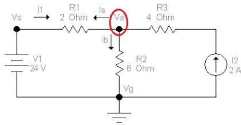
Gambar 11. Analisis Tegangan Node Va pada Rangkaian Listrik
