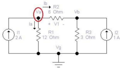
Gambar 6. Analisis Tegangan Node V_a Pada Rangkaian Listrik
