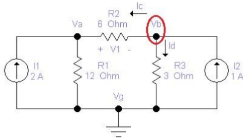
Gambar 7. Analisis Tegangan Node V_b Pada Rangkaian Listrik
