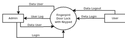
Gambar 1. Diagram blok sistem
