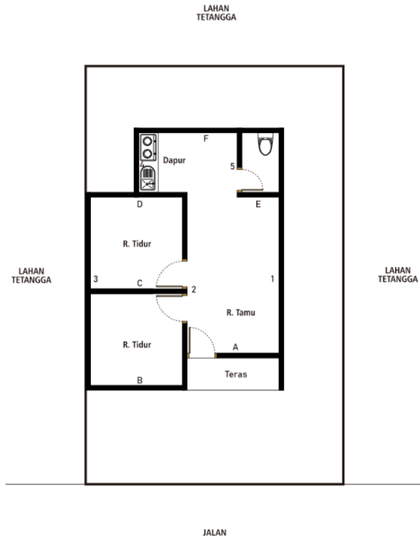
Gb.Denah Rumah untuk Pembuatan Maket Sumber : Dokumentasi Penulis, 2026
