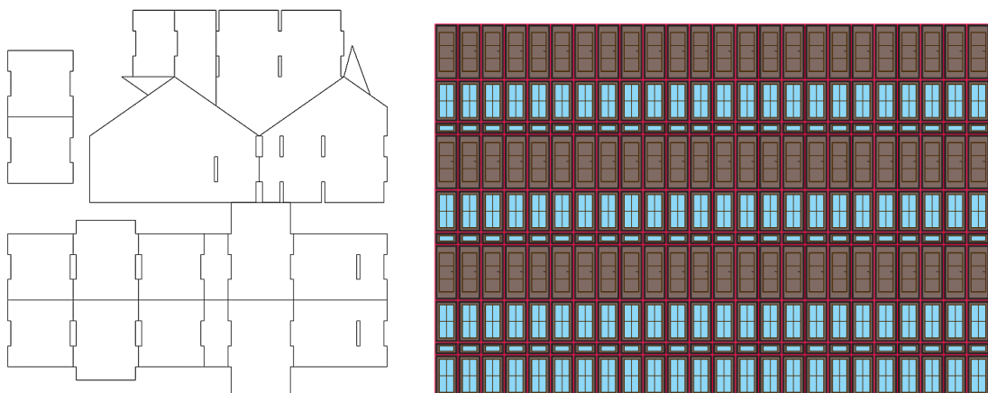
Gb.Pola Dinding dan Pintu Jendela untuk Maket Rumah Sumber : Dokumentasi Penulis, 2026
