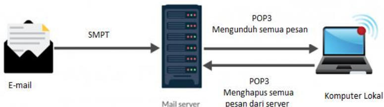
Gambar 9.2: Cara kerja POP 3
