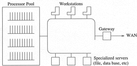
Gambar 2.6: Arsitektur Sistem Amoeba
