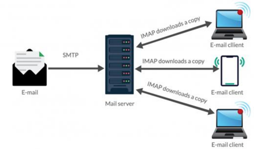
Gambar 9.3: Cara kerja IMAP
