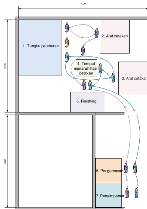
Gambar 3. Layout Awal Proses Produksi
